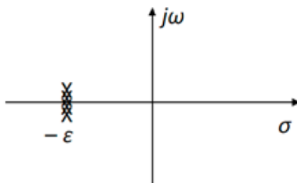
图 3 林氏低增益反馈极点模式
